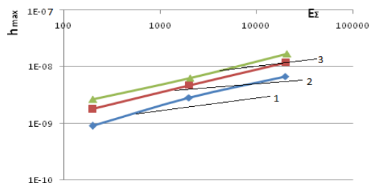
Рис. 3. Зависимость объема нанокластера (а), минимальной (б) и максимальной (в) глубины его залегания от энергии иона Y^+ ( 1 - z = 1 ; 2 - z = 2 и 3 - z = 3 ) при действии его на твердый сплав ВК8
