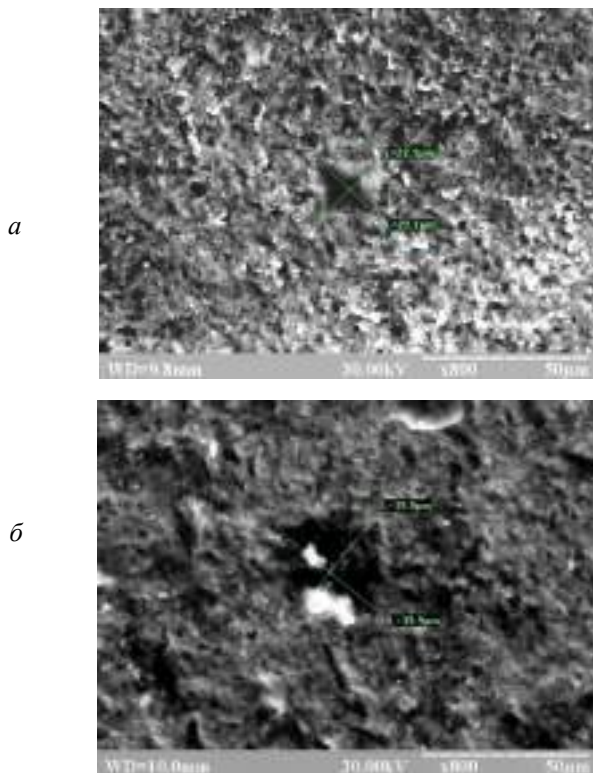
Рис. 2. Измерение твердости на твердосплавной пластине с наноструктурным покрытием Zr_{0,8}Hf_{0,2}N : а – марки IC 830; б – марки IC 808
