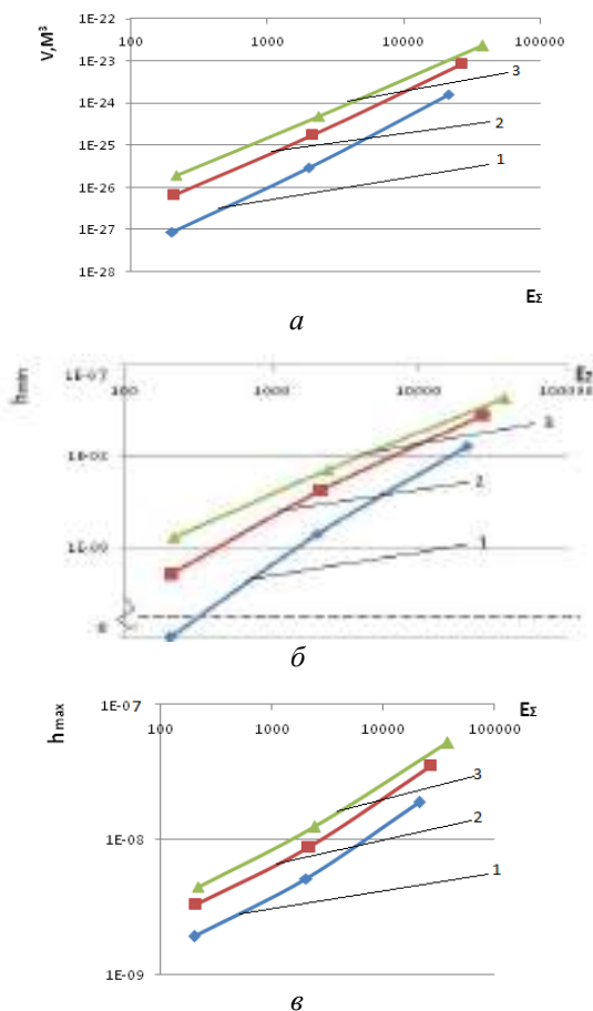
Рис. 1. Зависимость объема нанокластера ( a ), минимальной ( б ) и максимальной ( в ) глубины его залегания от энергии иона \text{B}^+ ( 1 - z = 1 ; 2 - z = 2 и 3 - z = 3 ) при действии его на твердый сплав ВК8
